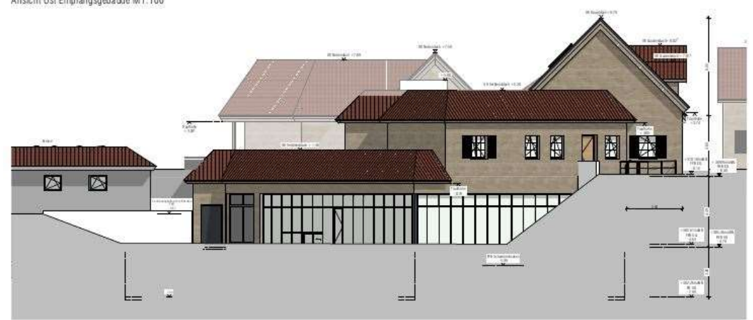
Ansicht Ost Empfangsgebäude M1:100
